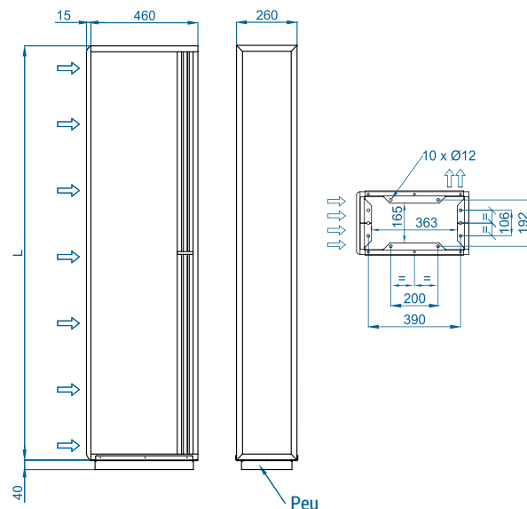
Instal·lació vertical
